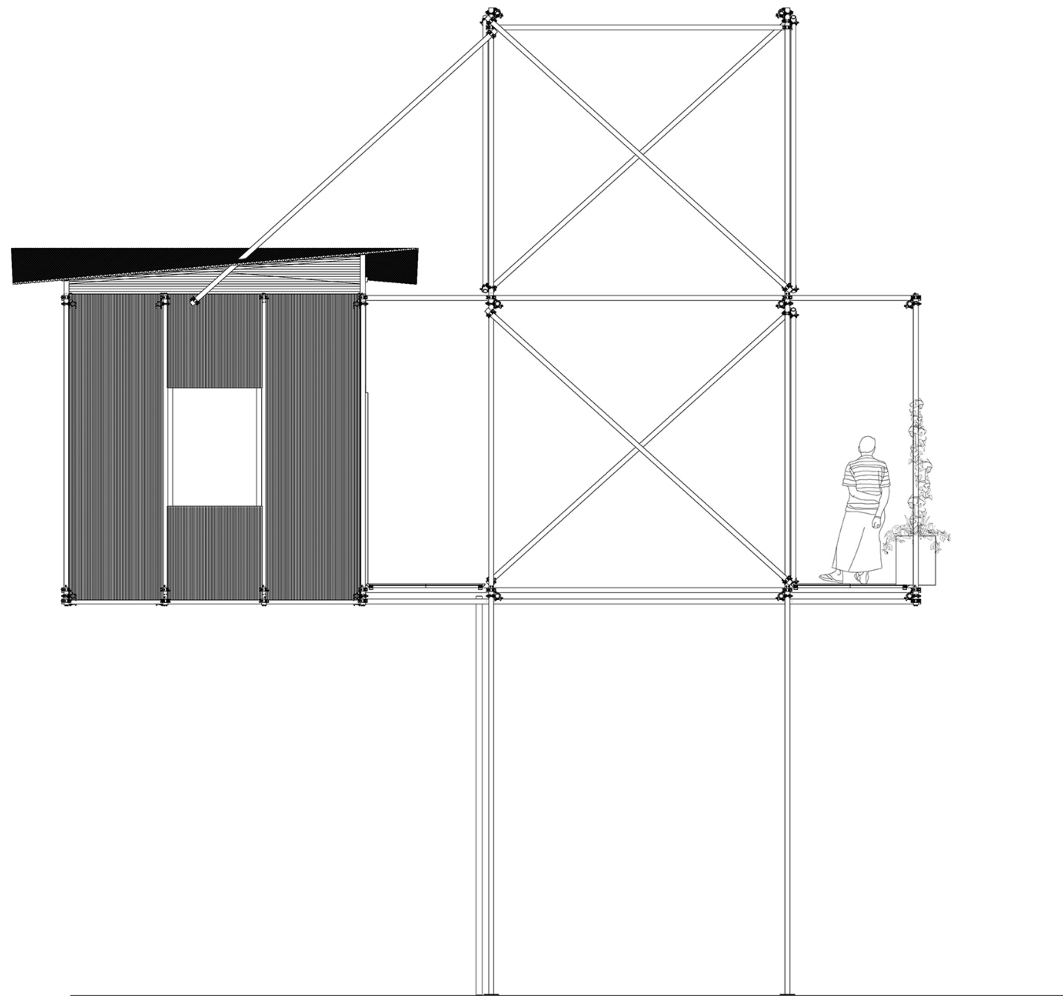
ELEVATION - C
