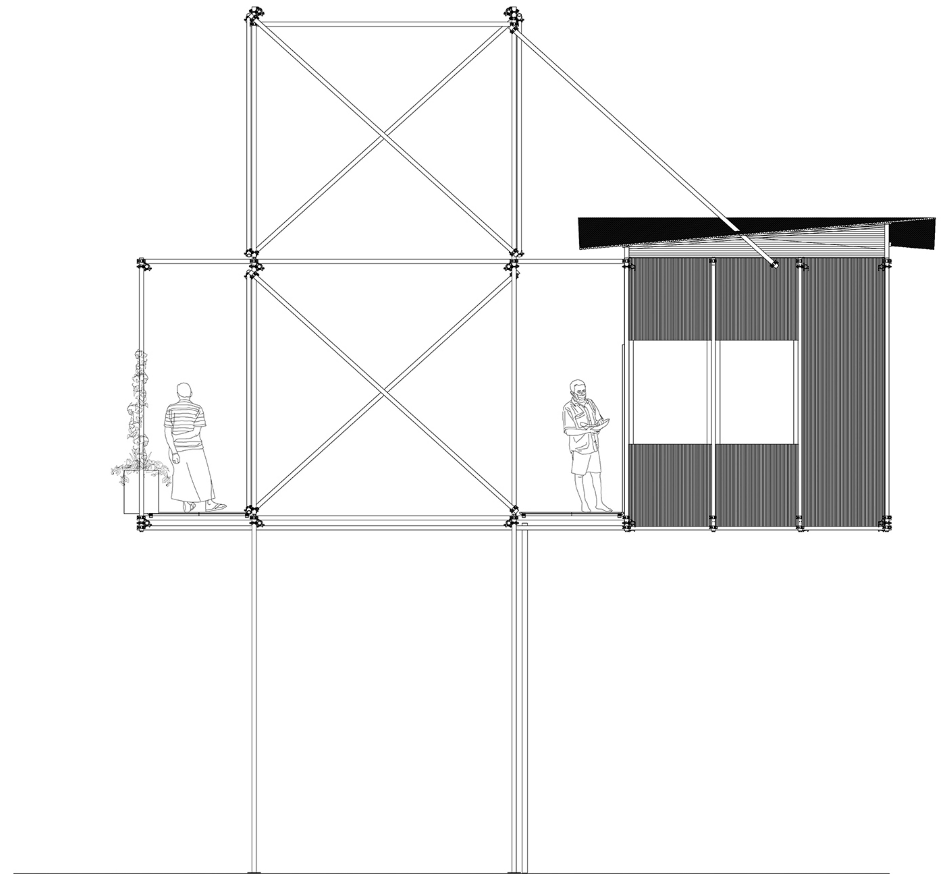
ELEVATION - D
